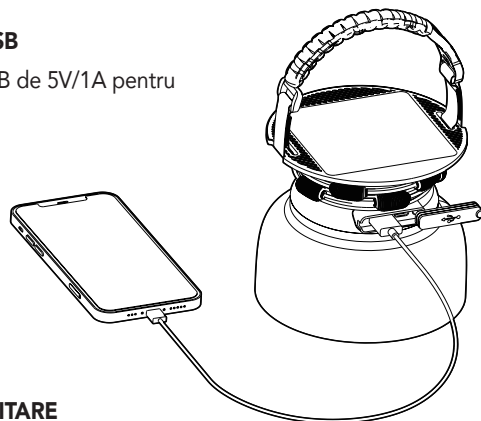
Încărcare prin cablu de tip USB-C
